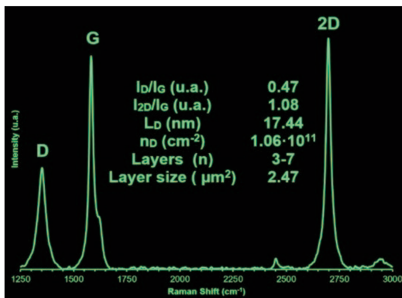
Figura 3. Espectro de Raman del grafeno obtenido.
